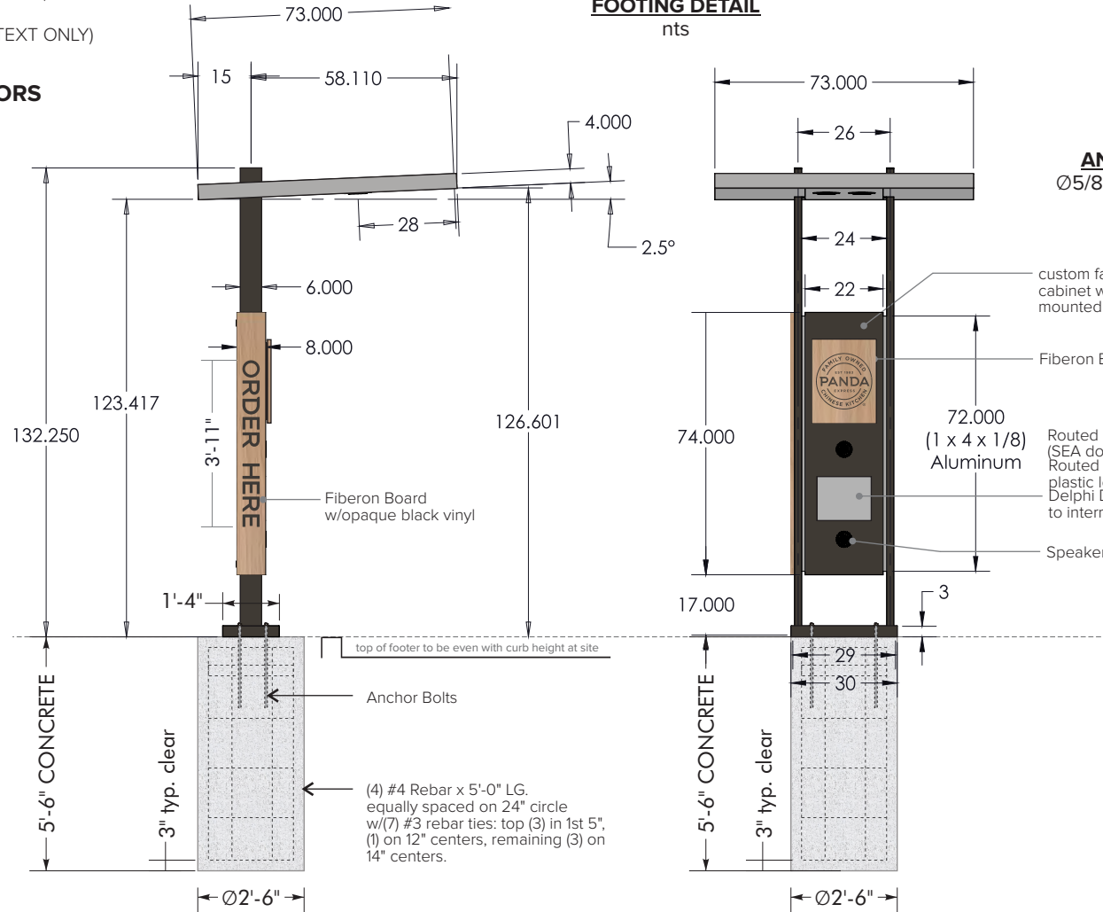
SCALE: 1/4" = 1'-0"
