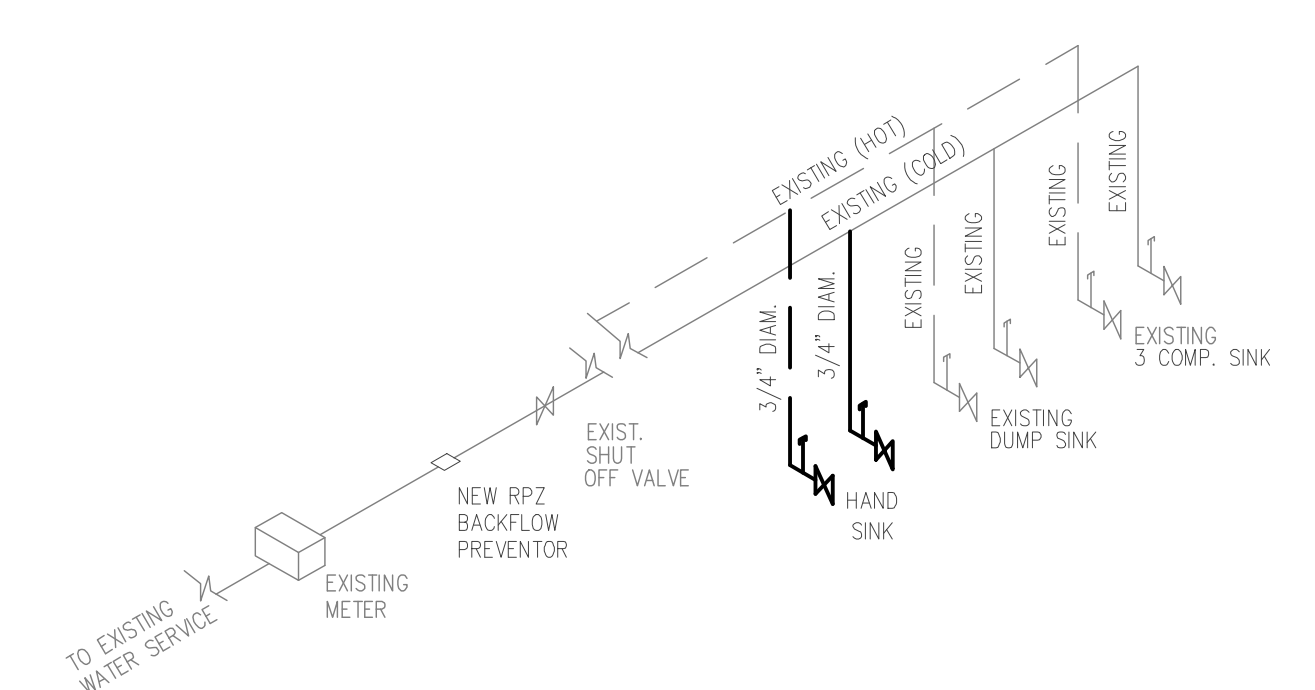
DOMESTIC WATER SCALE: N.T.S.
