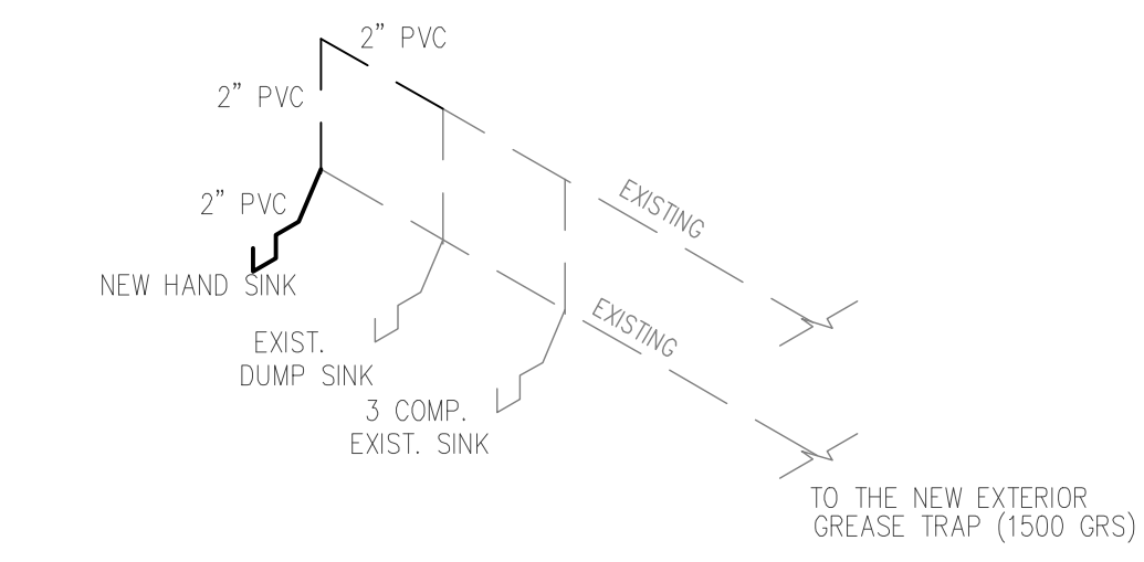
WASTE & VENT DIAGRAM SCALE: N.T.S.
