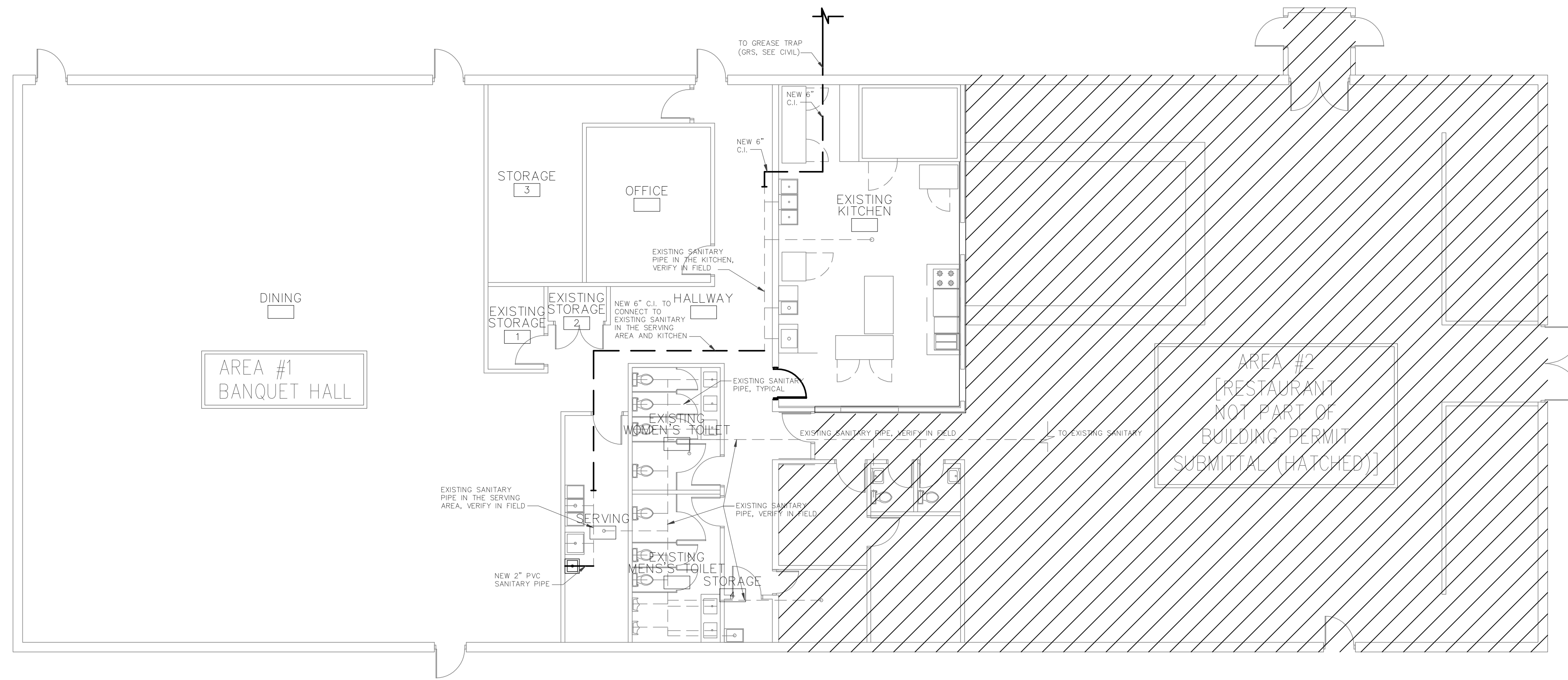
PLUMBING PLAN SCALE: 1/8" = 1'-0"
